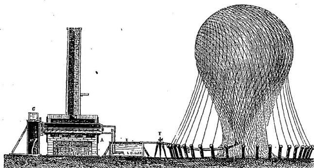
Appareil qui servait à préparer le gaz hydrogène, pour le remplissage de l'aérostat militaire l'Entreprenant.
